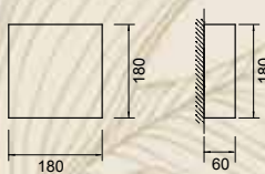
COLORVETRO 18 Led 17W - 230Vac - 3000K CE Peso / Weight 0,8 kg
