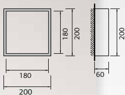
DIVETRO 18 WOOD Led 17W – 230Vac – 3000K CE Peso / Weight 0,9 kg
